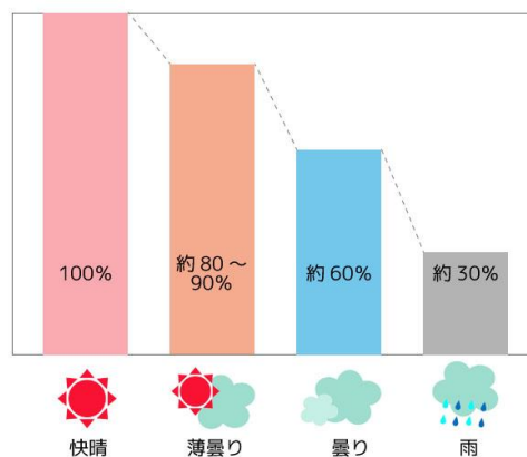
天気ごとの紫外線量の比率
